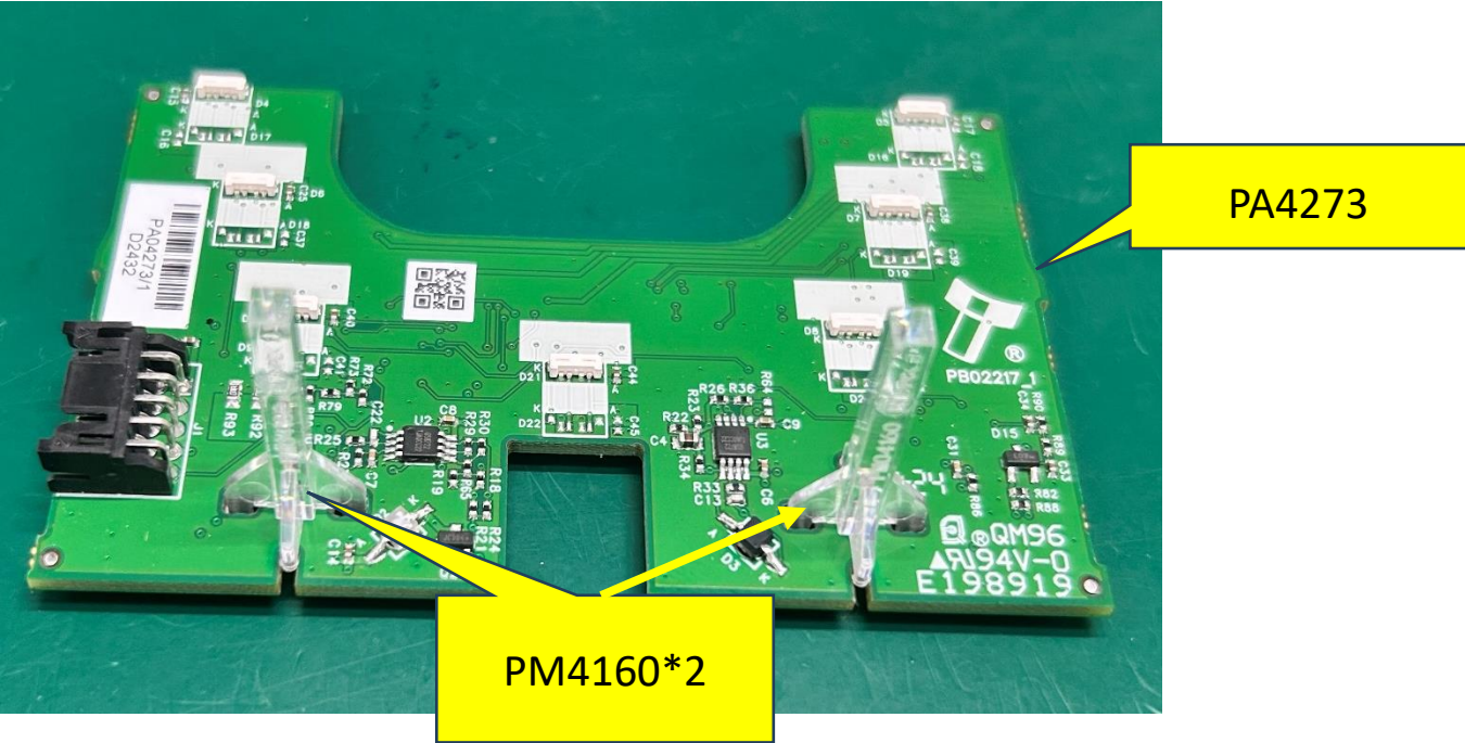
图一，将两个 PM4160 分别装入 PA4273 如图位置,注意有字方向朝边缘装入，两边卡扣扣合到位。
