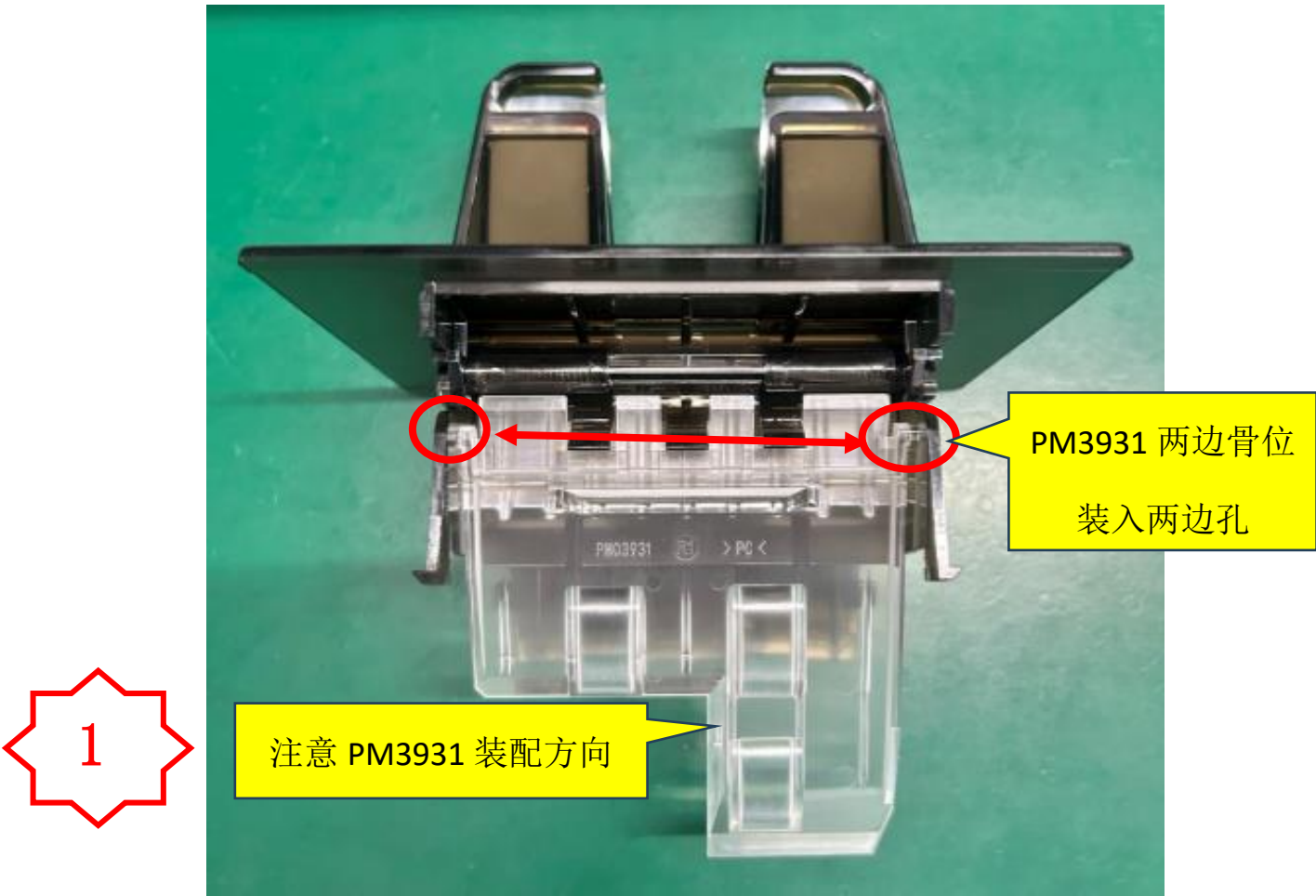
图一，将 PM3931 两边骨位装入 PA4354-3 两边孔,注意装配方向。
