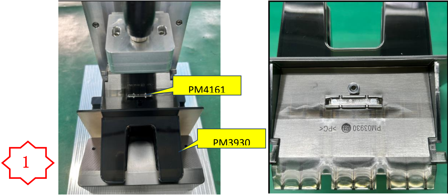
图一，将 PM3930 放入治具，再将 PM4161 放入导光柱槽位，有字朝上，PM4161 上 4 个骨位对 PM3930 上 4 槽位，用治具按压到位。
