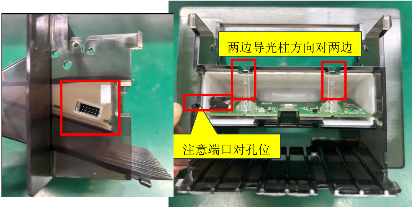
图二，检查两边扣装配到位，装配方向正确。
