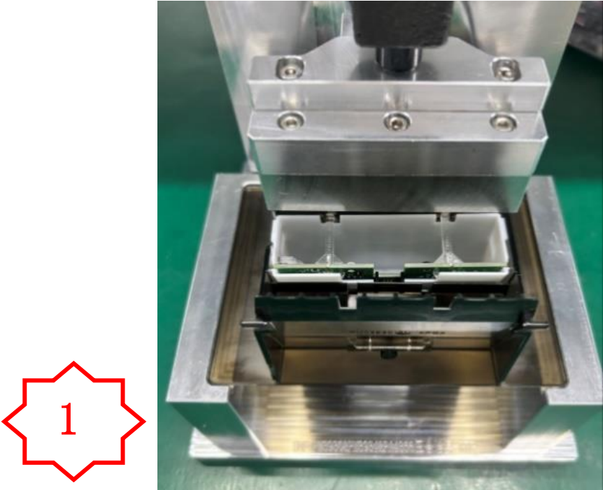
图一，将 PA4356 放入 PA4354-1，注意装入方向，再放入治具压合。
