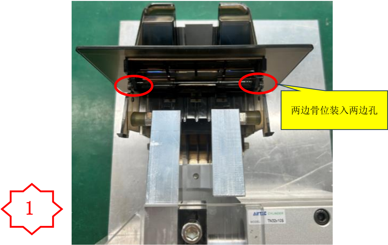
图一，将装好 PM3932 组件的物料放入气动治具，将左右撑开将 PM3932 两边骨位扣入 PM3930 两边孔位。
