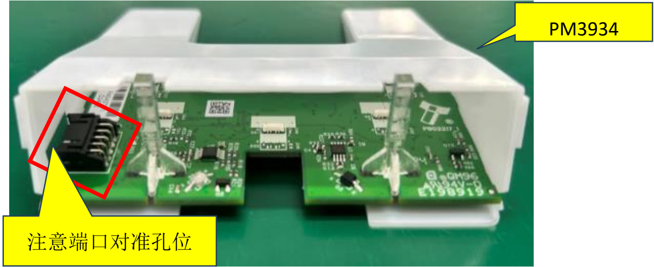
图一，将 PCB 板组件装入 PM3934，注意 PA4273 端口要对准 PM3934 孔位的方向装入。
