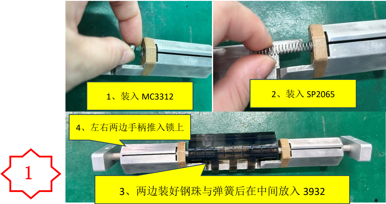
图一，先将两个 MC3312 装入治具两边孔，再在两边装入两个弹簧，完成后放入 PM3932,注意 PM3932 装配方向，确认物料都完成组装后将治具两边手柄锁上。
